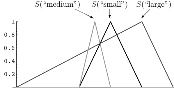
Fig. 4. A non-interpretable setting
